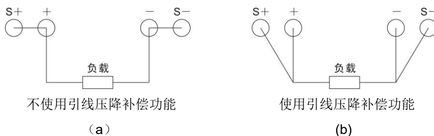
图 1-1 输出接线
