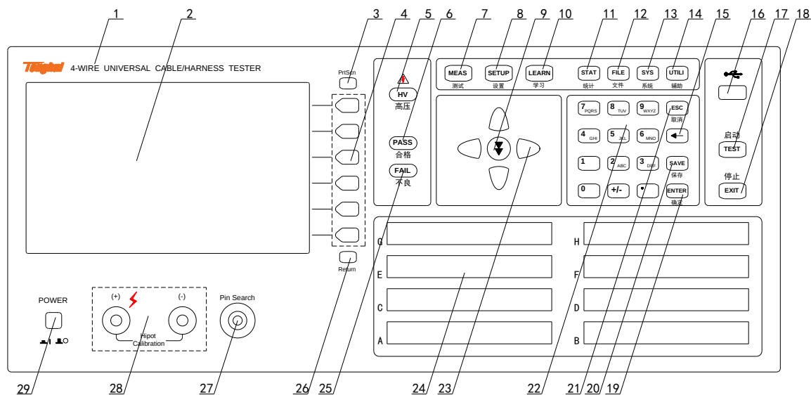
图 2-1. 前面板说明
