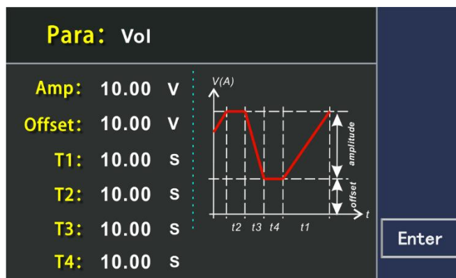
图 3-32 输出梯形波
