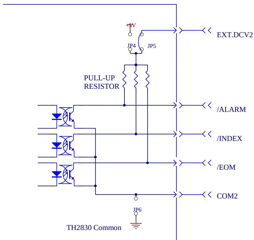
控制信号输入电路
