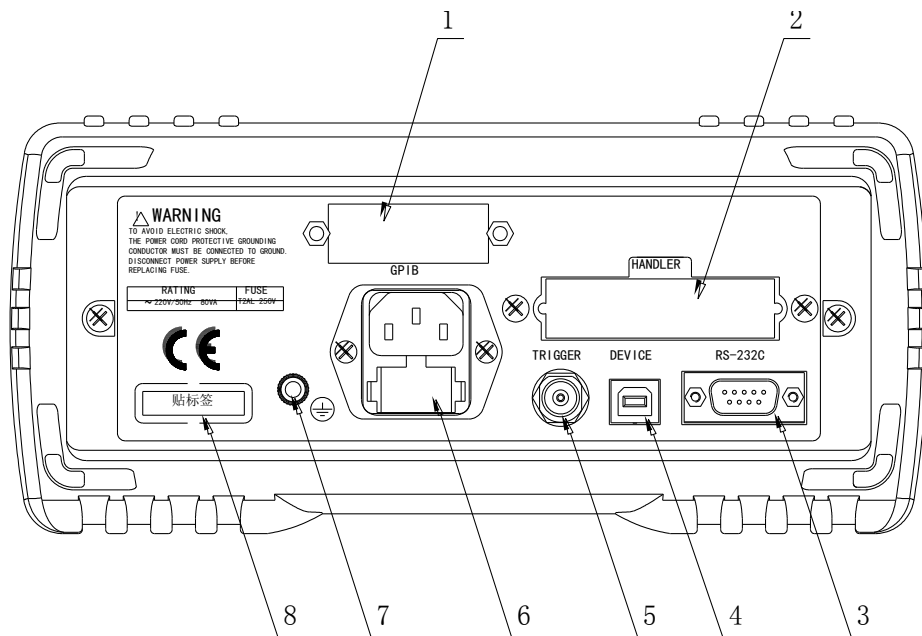
图 2-2. 后面板说明
