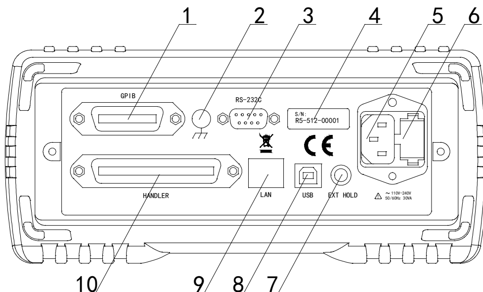
图 2-2 后面板说明
