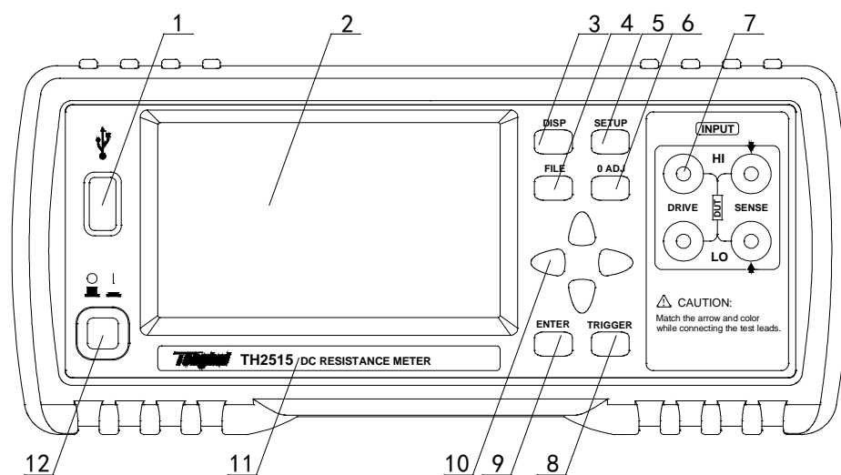
图 2-1 前面板说明
