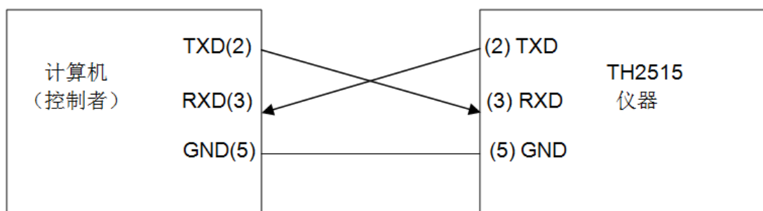
图 6-2 计算机与仪器连接示意图
