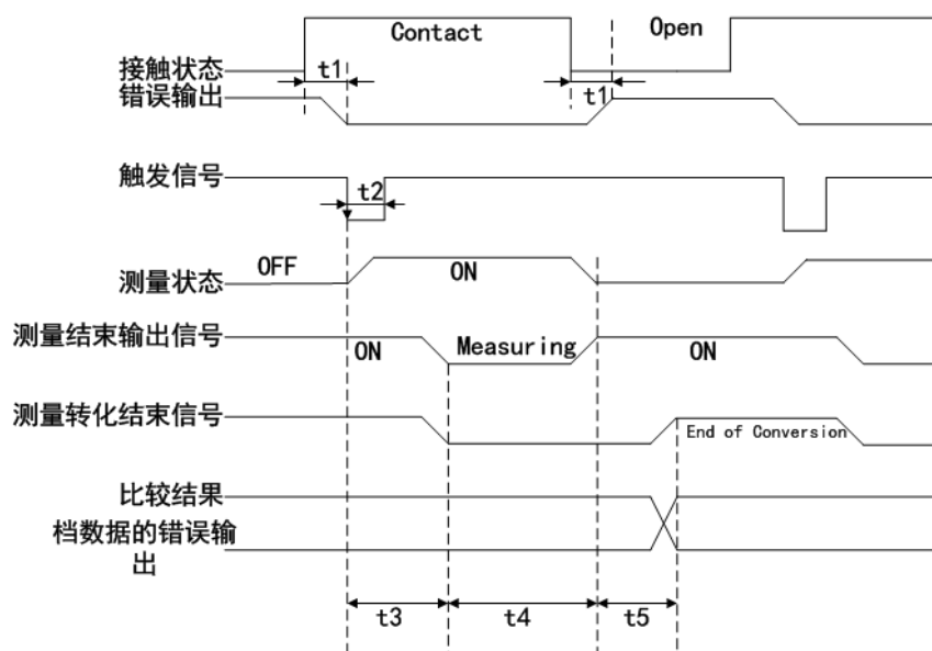
图 3-20 外部触发时序
