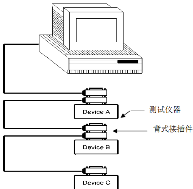
图 6-4 双背式接插件叠加
