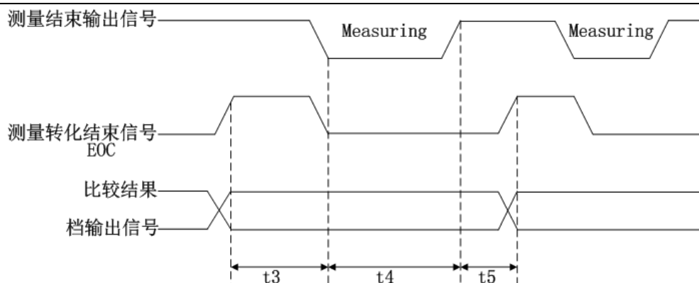
图 3-21 内部触发时序
