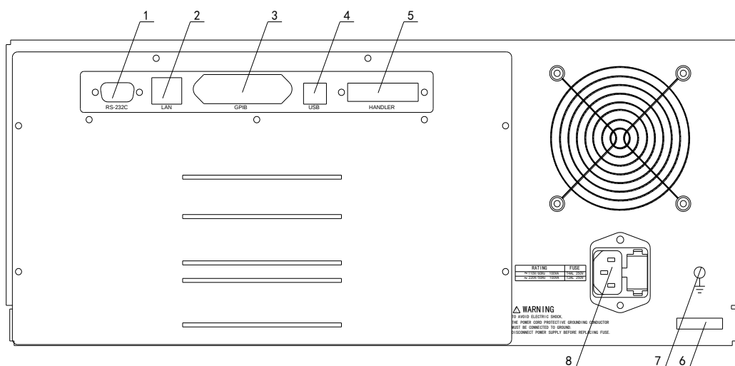
图 2-2. 后面板说明
