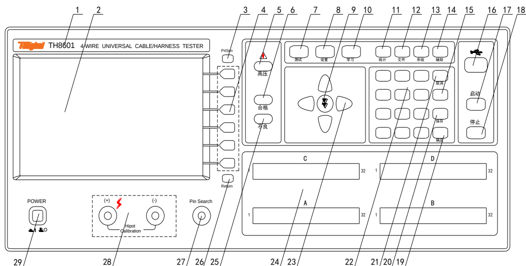
图 2-1. 前面板说明
