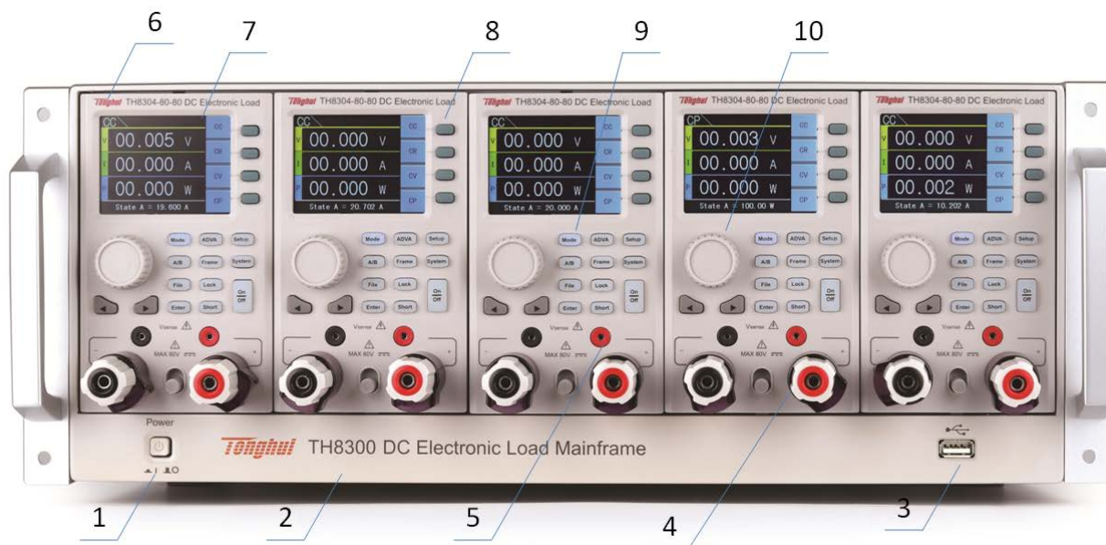
图 2-1 前面板
