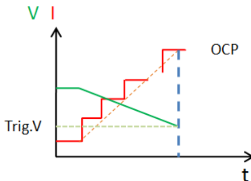
图 3-8 OCPT 模式
