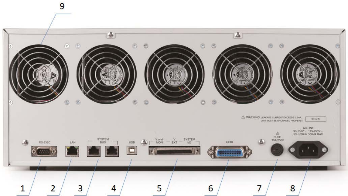
图 2-2 后面板
