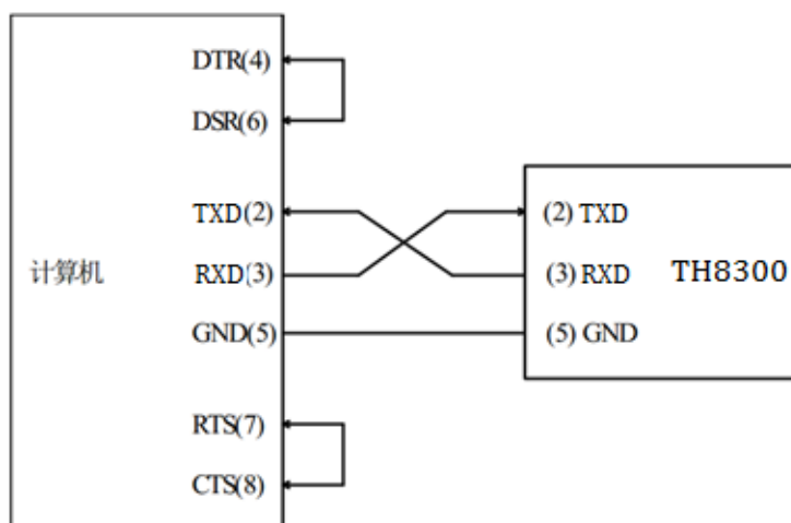
图 6-2 RS-232 接线图
