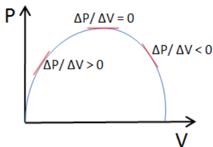
图 3-7 MPPT 模式
