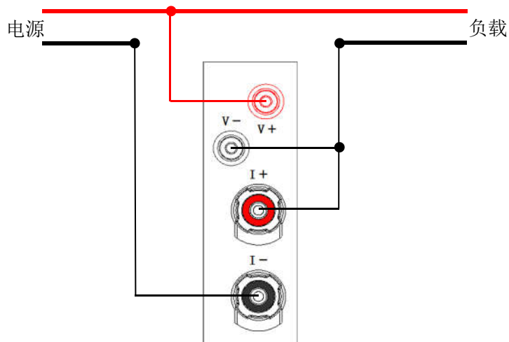
（图 8-2 电流表内接法--适用于大电流接法）
