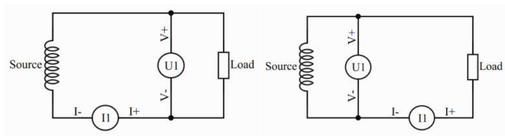
图 8-3 电流表内接(左)，电流表外接(右)—原理示意图
