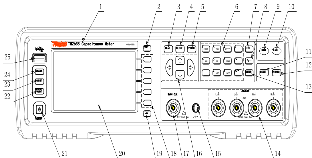
图 2-1 前面板
