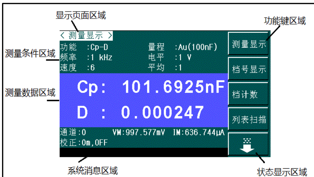
图 2-3 屏幕显示
