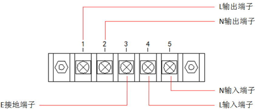
图 1-1 接线示意图
