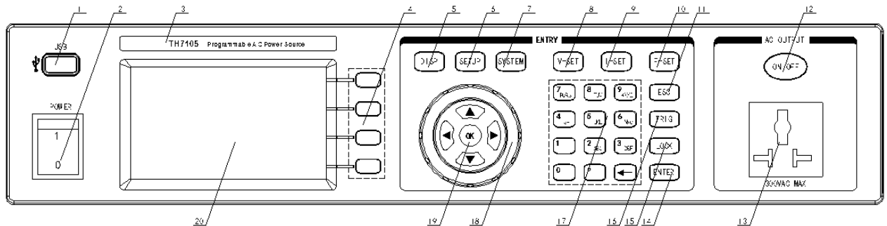
图 2-1 前面板
