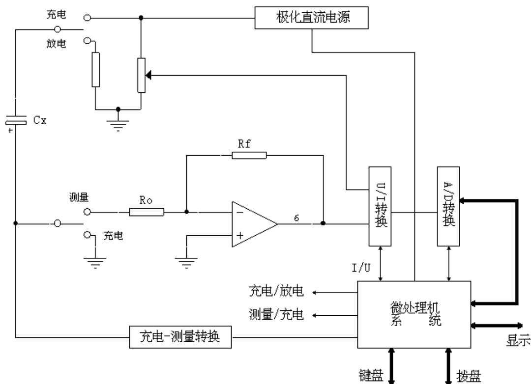
图 2 仪器框图
