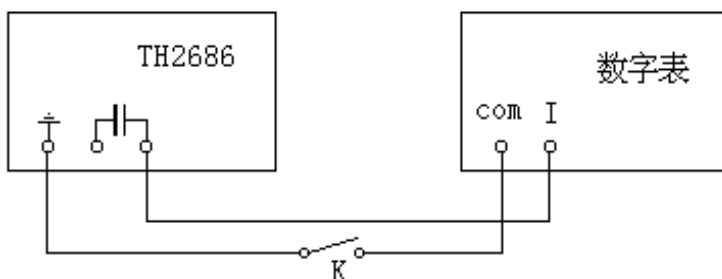
图 4 最大充电电流的校准与检验
