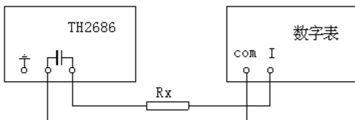
图 5 漏电流的校准与检验
