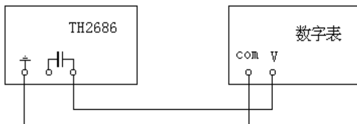
图 3 直流极化电压的检验和校准
