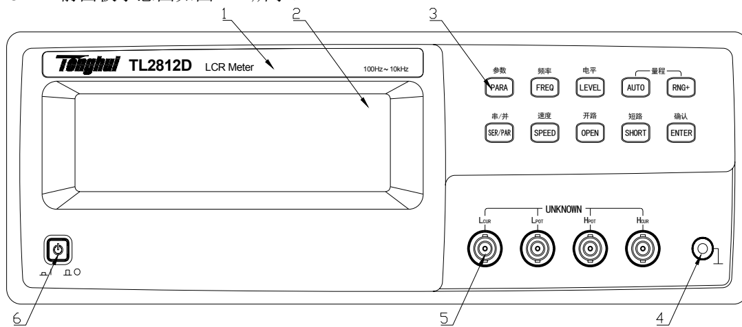
图 2-1. 前面板
