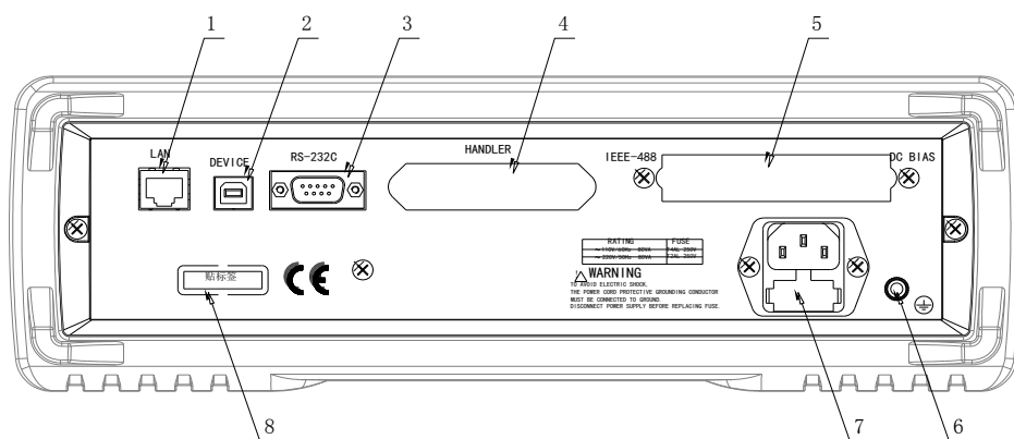
图 2-2. 后面板说明
