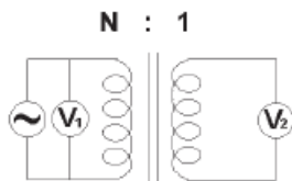
图 5—18 电压比法直接测量匝比
