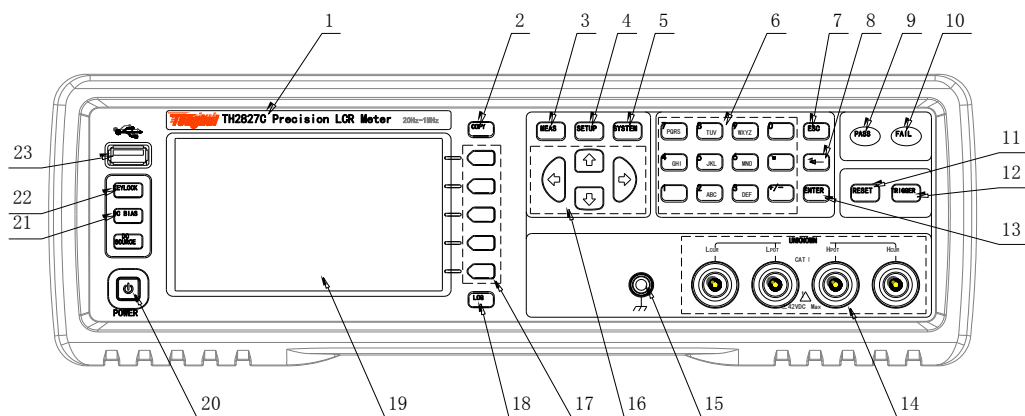
图 2-1. 前面板说明
