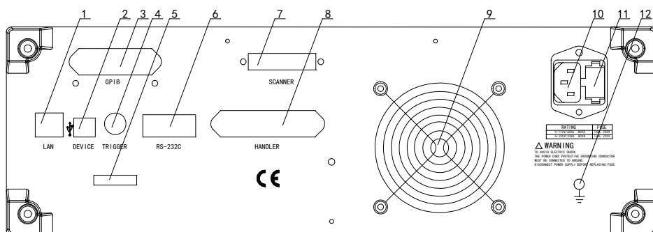
图 2-2. 后面板说明
