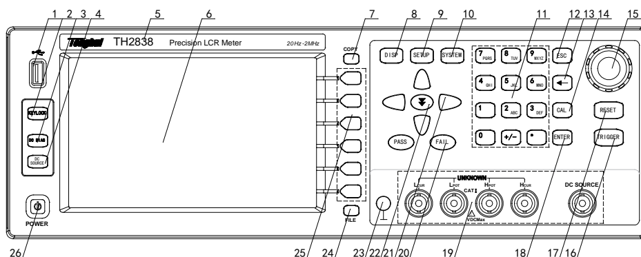
图 2-1. 前面板说明
